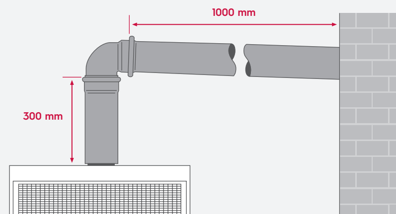
Disposizione di misurazione (come previsto dalla norma)
