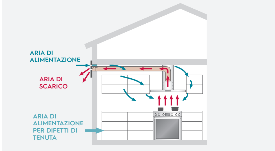
Rappresentazione schematica: cassetta a muro per aria di scarico e di alimentazione
