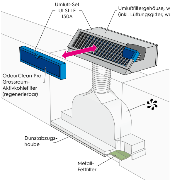
UL SLLF 150A passend zu Oberschrank ohne Blende
