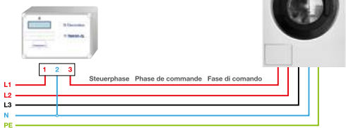
Schema d'allacciamento
