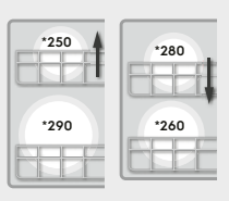
Taille maximale des assiettes lave-vaisselle norme Euro avec 13 couverts standard (*hauteur standard)
