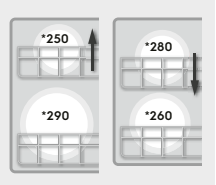
Dimensioni massime dei piatti Lavastoviglie EURO-Norma con 13 coperti standard (*altezza STD)
