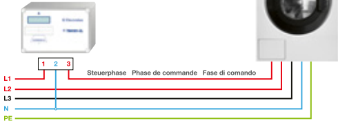
Schema d’allacciamento
