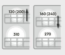
Dimensione max. piatti 45 cm Lavastoviglie con cassetto portaposate e 10 coperti (senza cassetto portaposate e 9 coperti)
