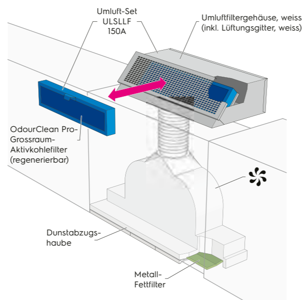
UL5LLF150A passend zu Oberschrank ohne Blende
