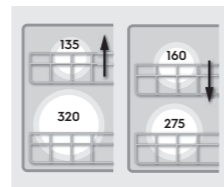
Maximale Tellergrössen SMS-Norm-Geschirrspüler mit 12 Massgedecken
