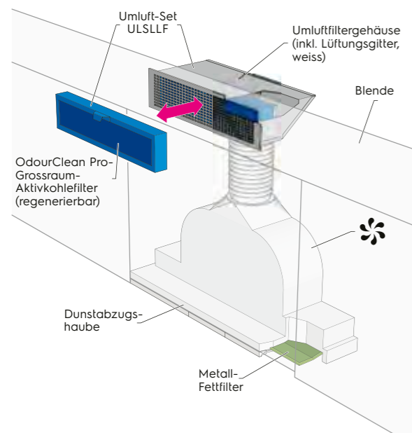
UL5LLF I UL5LLF125 passend zu Oberschrank mit Blende (Ausschnittmass 115 x 510 mm)
