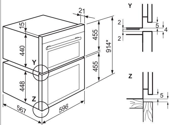
Cave à vin + Four encastrable Compact 45 WK4PL10 + EB4...
