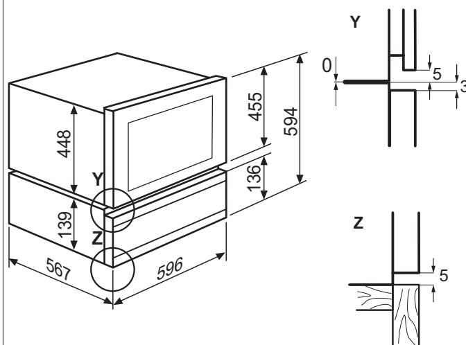
Tiroir de mise sous vide/Tiroir des accessoires + Cave à vin VAC140PL(V)/ZS140GL + WK4PL10
