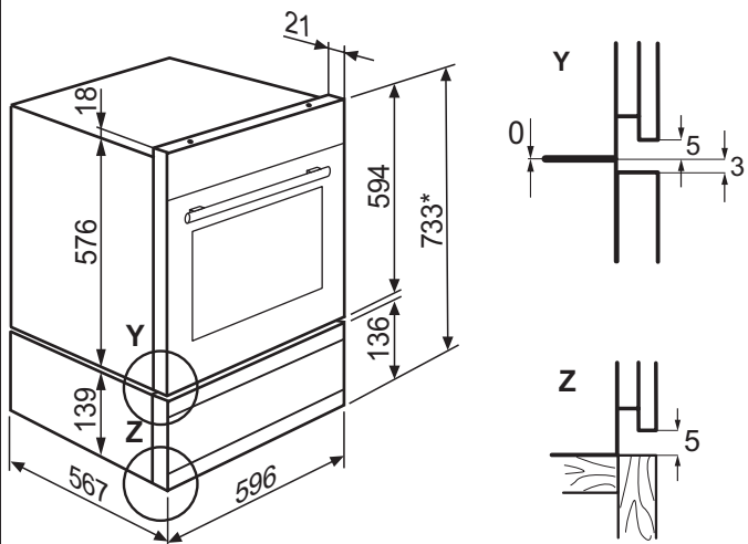
Tiroir encastré + four encastrable ZS140GL... + EB6...
