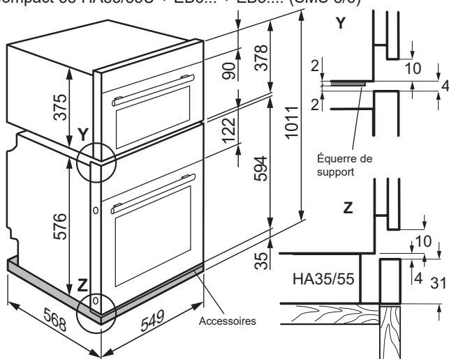
Adaptateur de hauteur + four encastrable court + four encastrable Compact 38 HA35/55U + EB6... + EB3... (SMS 8/6)
