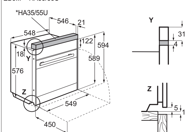
Forno da incasso piccolo + adattatore di altezza EB6... + HA35/55U
