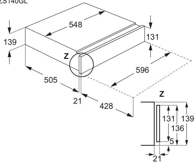
Cassetto accessori ZS140GL
