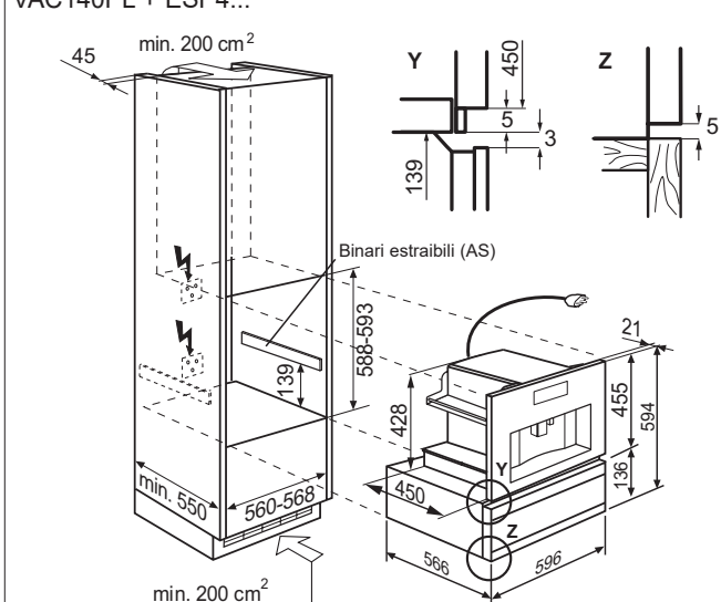
Cassetto per la conservazione sottovuoto + Macchina per caffè VAC140PL + ESP4...
