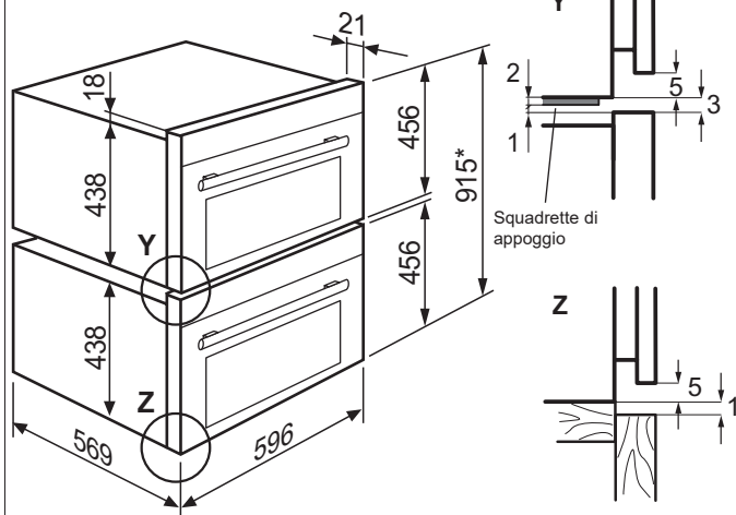
Forno da incasso Compact da 45 + forno da incasso Compact da 45 EB4... + EB4...
