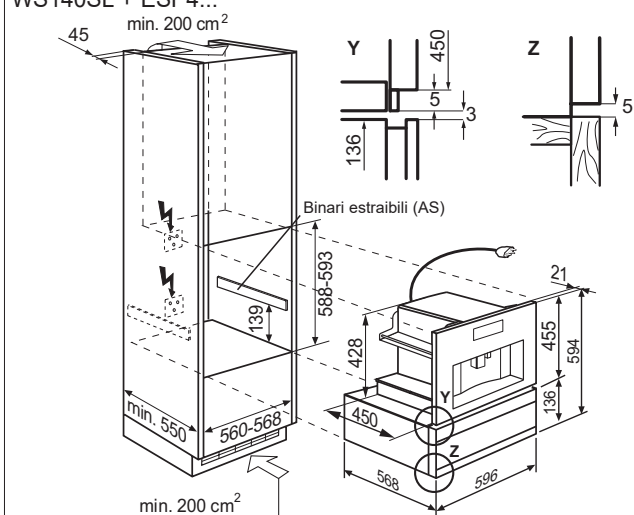
Cassetto scaldavivande + Macchina per caffè WS140SL + ESP4...
