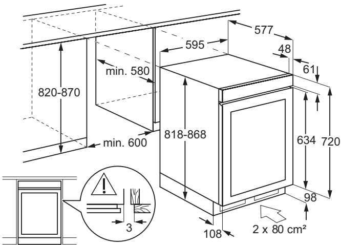
Armadio per vini sottobanco WKU60DSP
