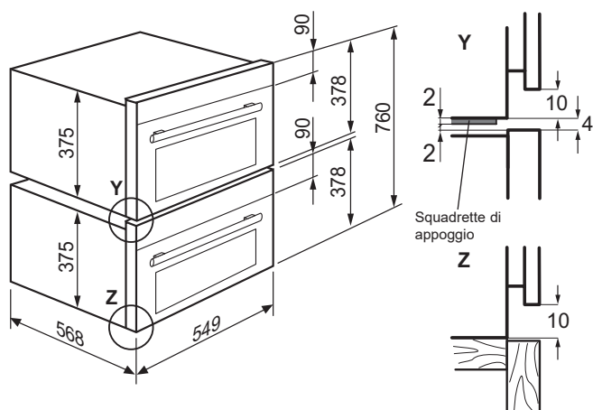
Forno da incasso Compact da 38 + forno da incasso Compact da 38 EB3... + EB3... (SMS 6/6)
