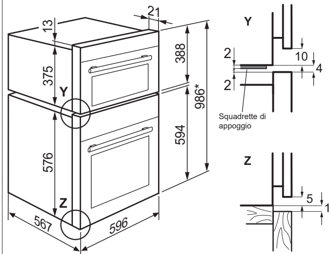
Forno da incasso + forno da incasso Compact da 38 EB6... + EB3...
