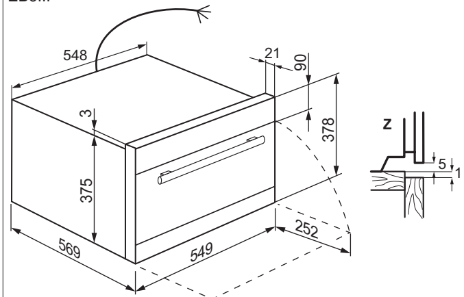
Forno da incasso Compact da 38 EB3...
