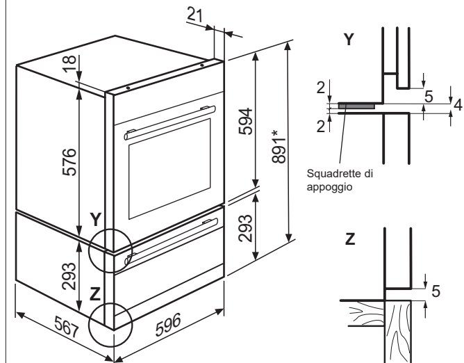
Cassetto scaldavivande + forno da incasso WS290SL... + EB6...
