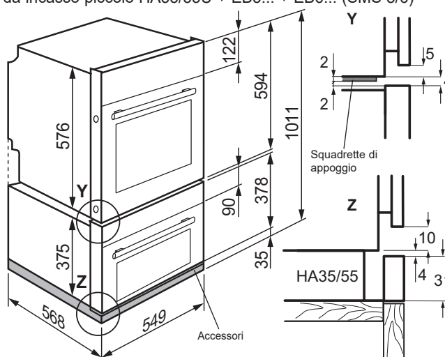
Adattatore di altezza + forno da incasso Compact da 38 + forno da incasso piccolo HA35/55U + EB3... + EB6... (SMS 8/6)
