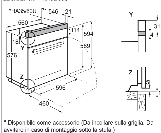
Forno da incasso/cucina da incasso + adattatore di altezza EB6.../EH6... + HA35/60U
