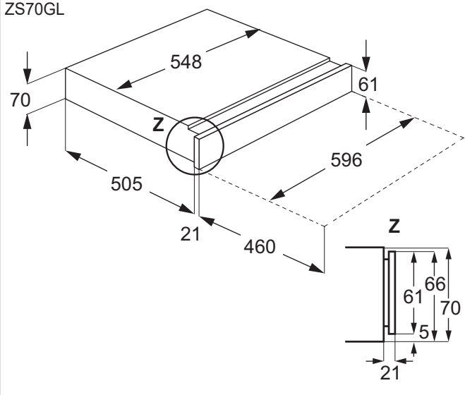
Cassetto accessori ZS70GL
