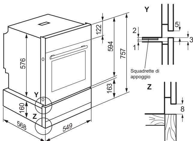
Cassetto scaldavivande + forno da incasso piccolo WS16SL + EB6... (SMS 6/6)
