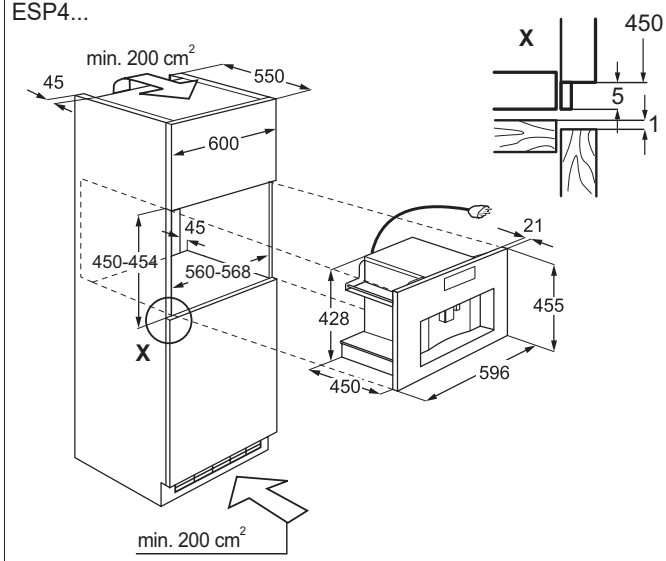
Cassetto scaldavivande + Macchina per caffè WS140SL + ESP4...
