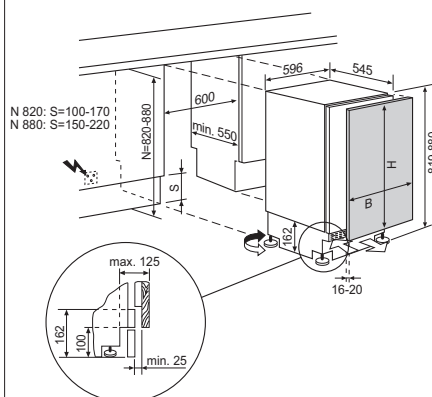
UK120S / UG0985 (SMS) Frontale avvitato sulla porta dell'apparecchio
