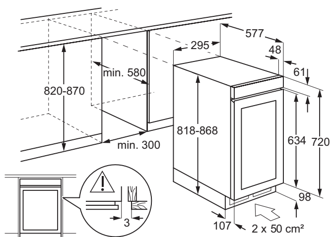
Armadio per vini sottobanco WKU30SSP
