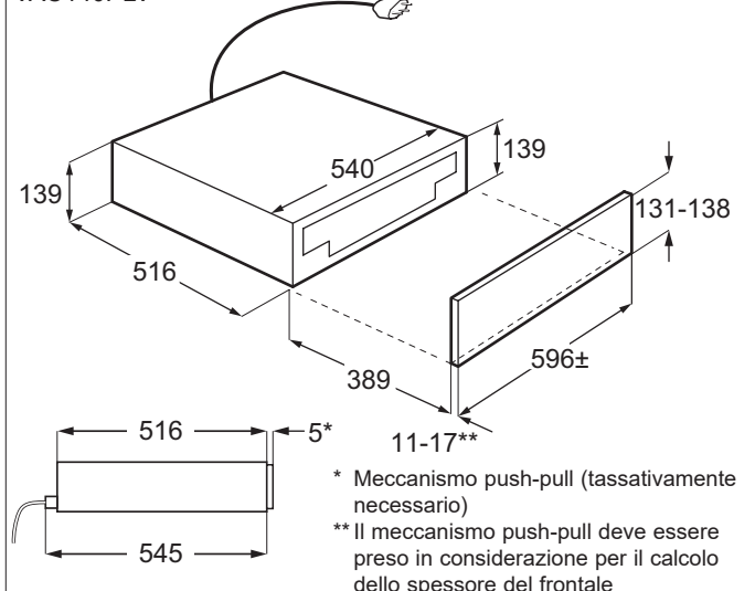
Cassetto per la conservazione sottovuoto VAC140PLV
