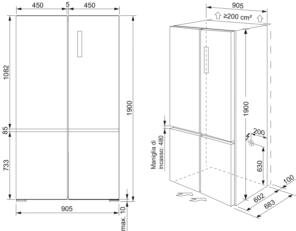
MD530NOCN (senza collegamento all'acqua)
