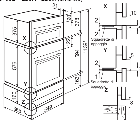
Cassetto scaldavivande + forno da incasso piccolo + forno da incasso Compact da 38 WS16SL + EB6... + EB3... (SMS 9/6)
