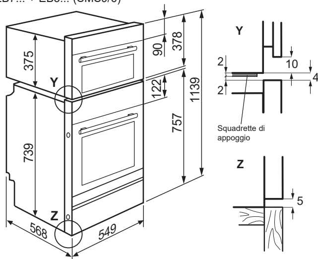
Forno da incasso + forno da incasso Compact da 38 EB7... + EB3... (SMS9/6)
