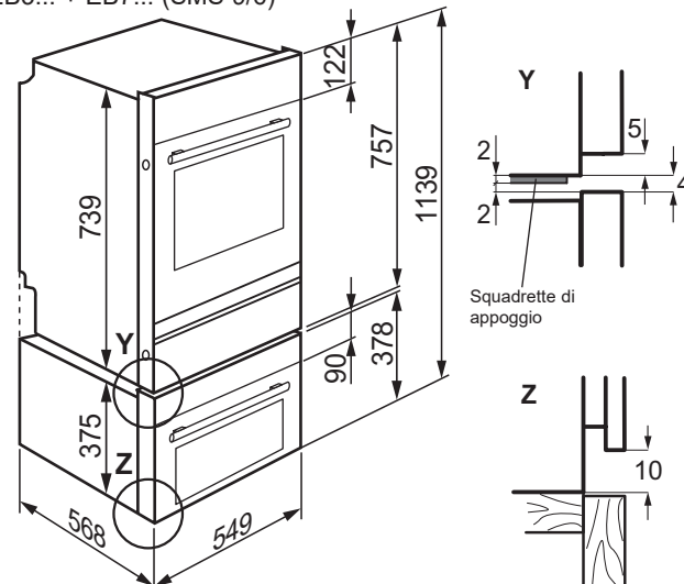
Forno da incasso Compact da 38 + forno da incasso EB3... + EB7... (SMS 9/6)
